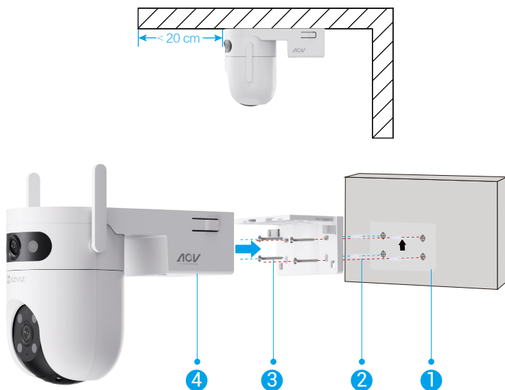
Fig. 2 Montaggio a parete
